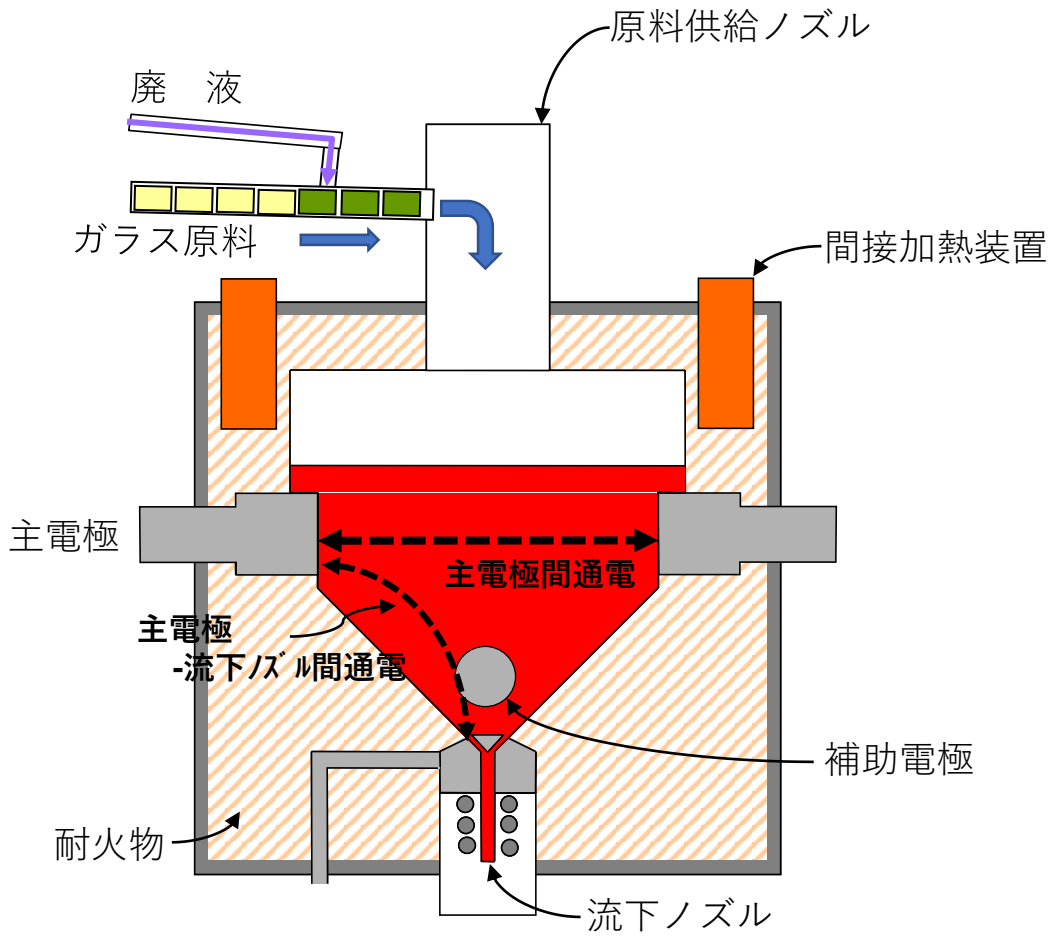
溶融炉断面
