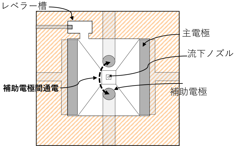
溶融炉平面
